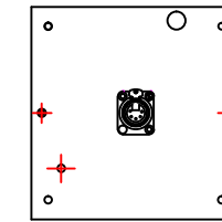
DMX-OUT-1回路 (NWC-4100D)
