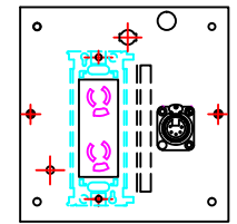
15AW-回路+DMX-OUT (NWC-4115D)
