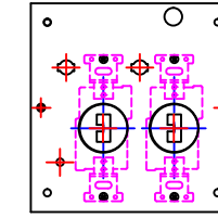
C型20A-2回路 (NWC-42200)
