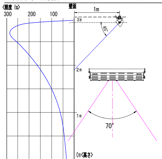
1灯点灯時の照度表 (NBF-2611K~2611W)
